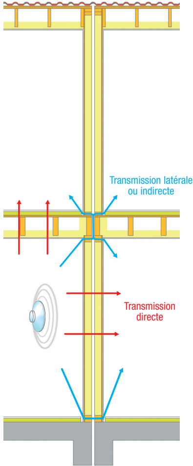
Transmissions directes et latérales / indirectes du bruit aérien d'une maison mitoyenne
